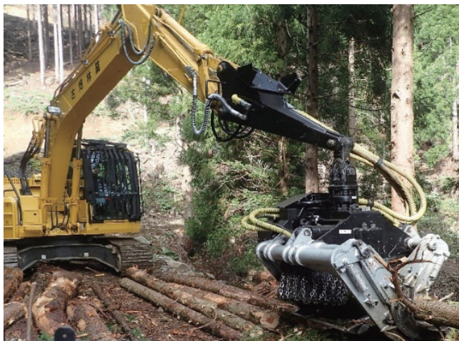
造材作業中
