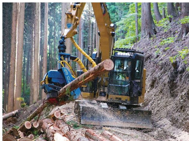
ハーベスタ稼働中
